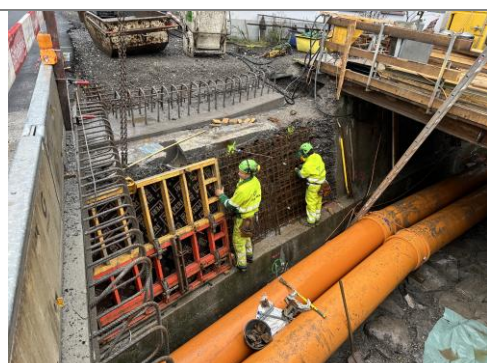
23.10.2025 / Hüribach – Schalung und Bewehrung Ufermauer
