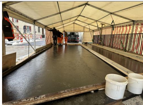
24.11.2025 / Hüribach – Einbau Gussasphalt Fahrs pur Schwyz
