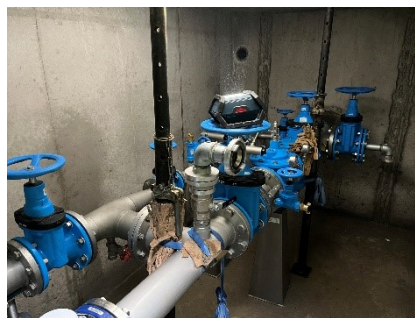
Druckreduzierschacht Zwingsbrücke
